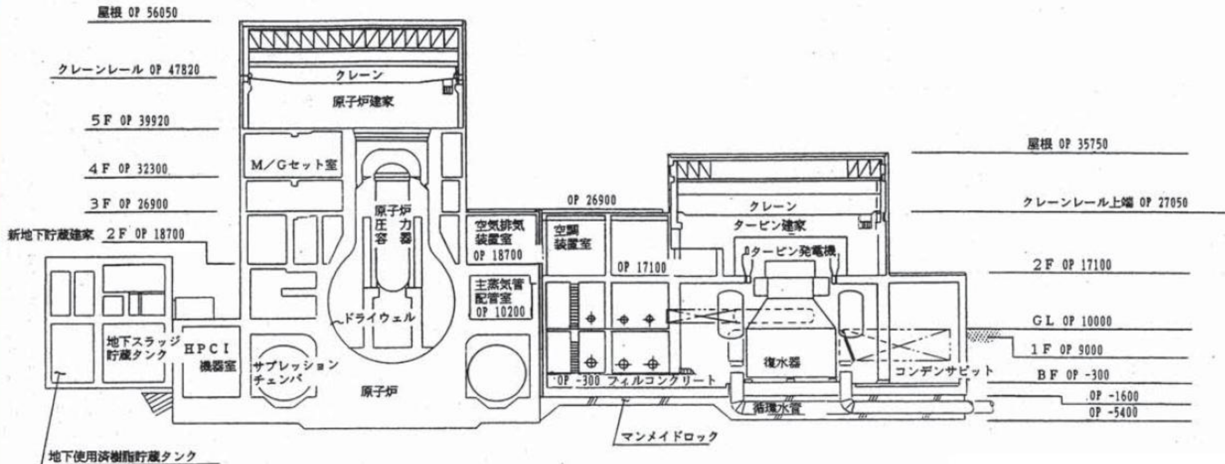
A-A断面
