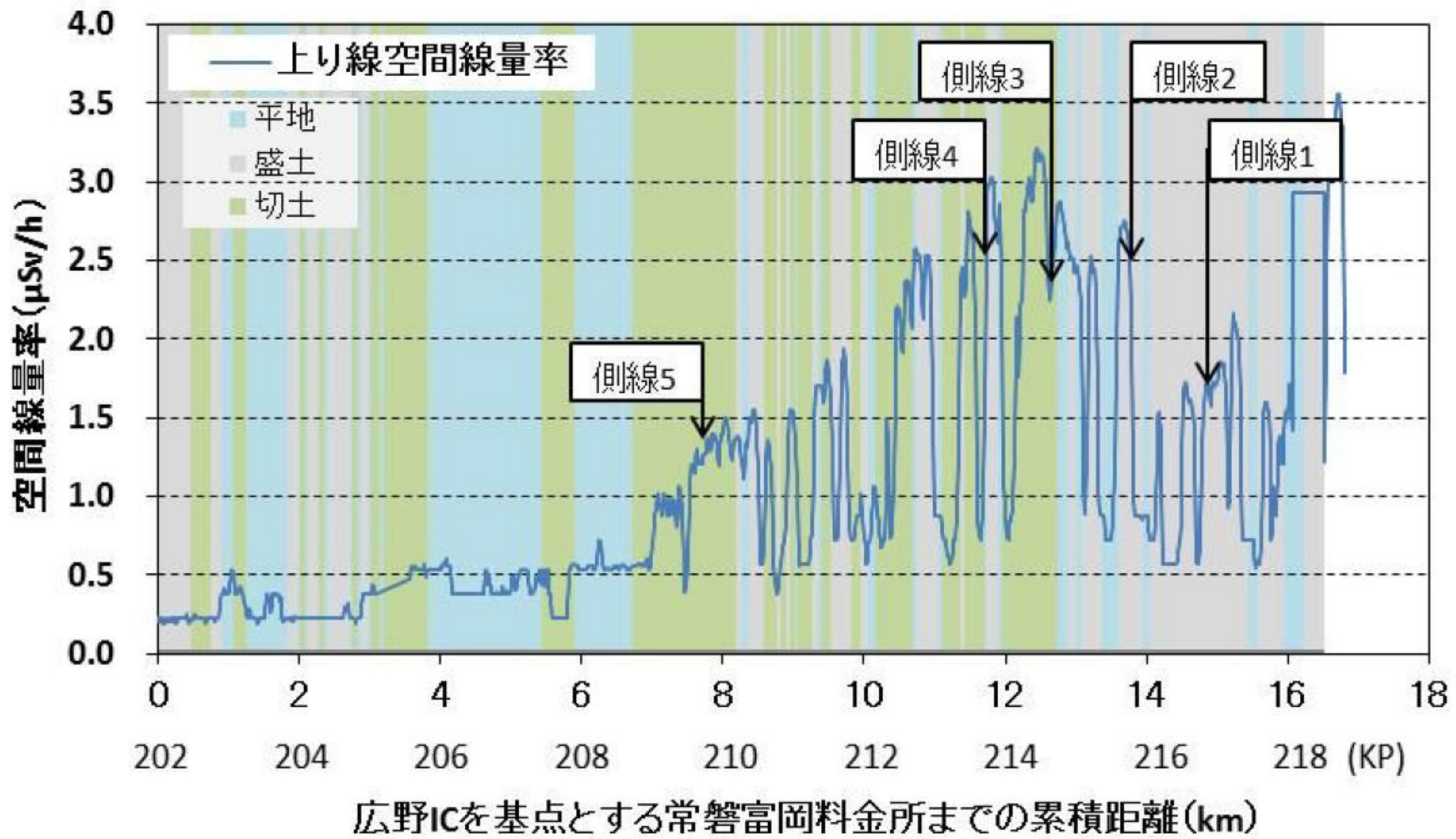
図 5-7 道路構造形式と空間線量率の関係 (上り線)
