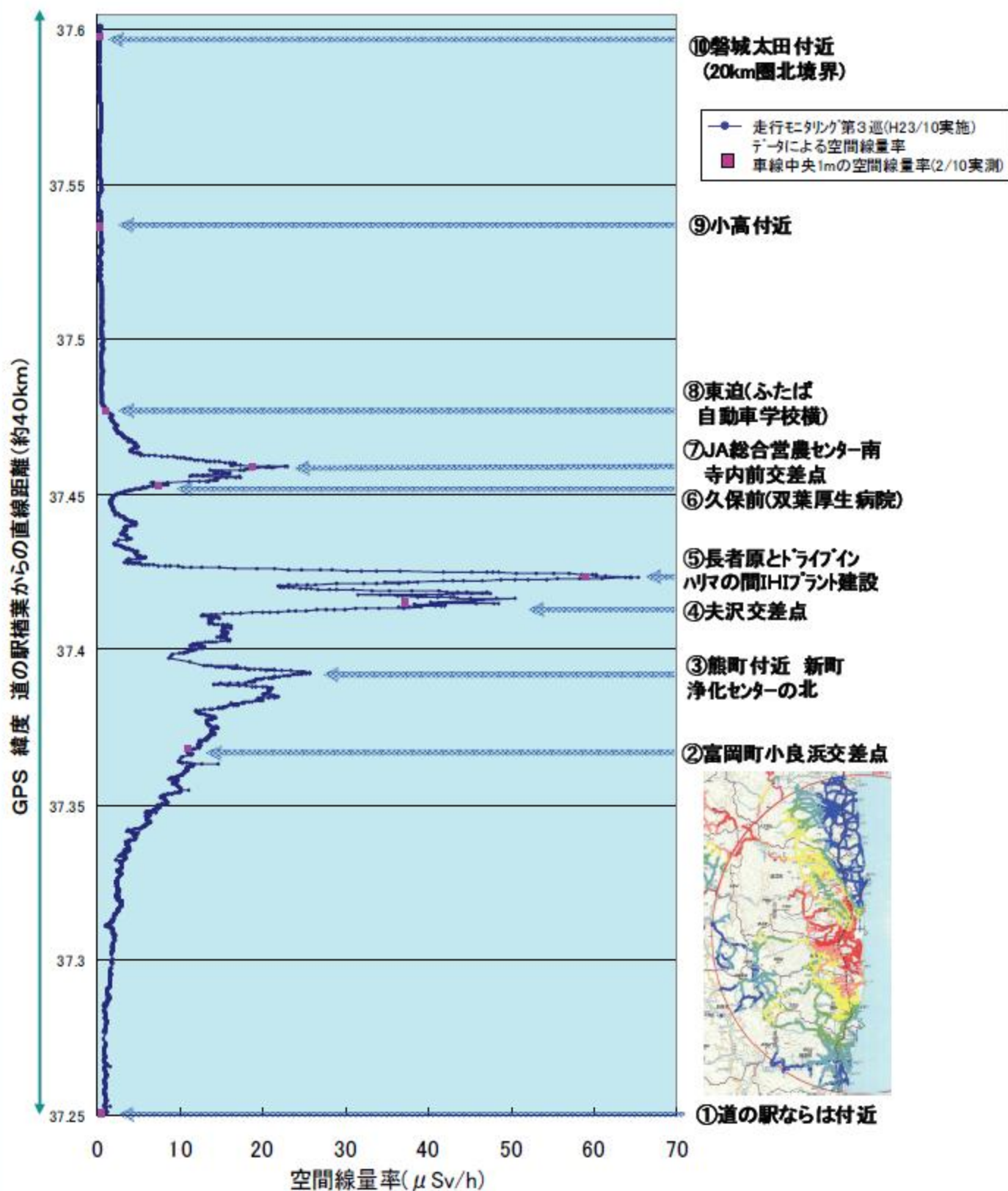
図6 国道6号のGPS実測データから走行モニタリング第3巡データより抽出した空間線量率分布とサンプリングポイントにおける車線中央1mの空間線量率の実測値
